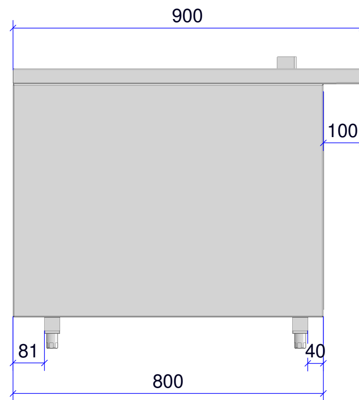
Converge® Multi-Cook Oven Laag Onderstel Uitsparing Voor Warmhoudlade 500-2D / 2DI EN 2X 6 REGALEN (KLP-BASE-CMC2REG)
