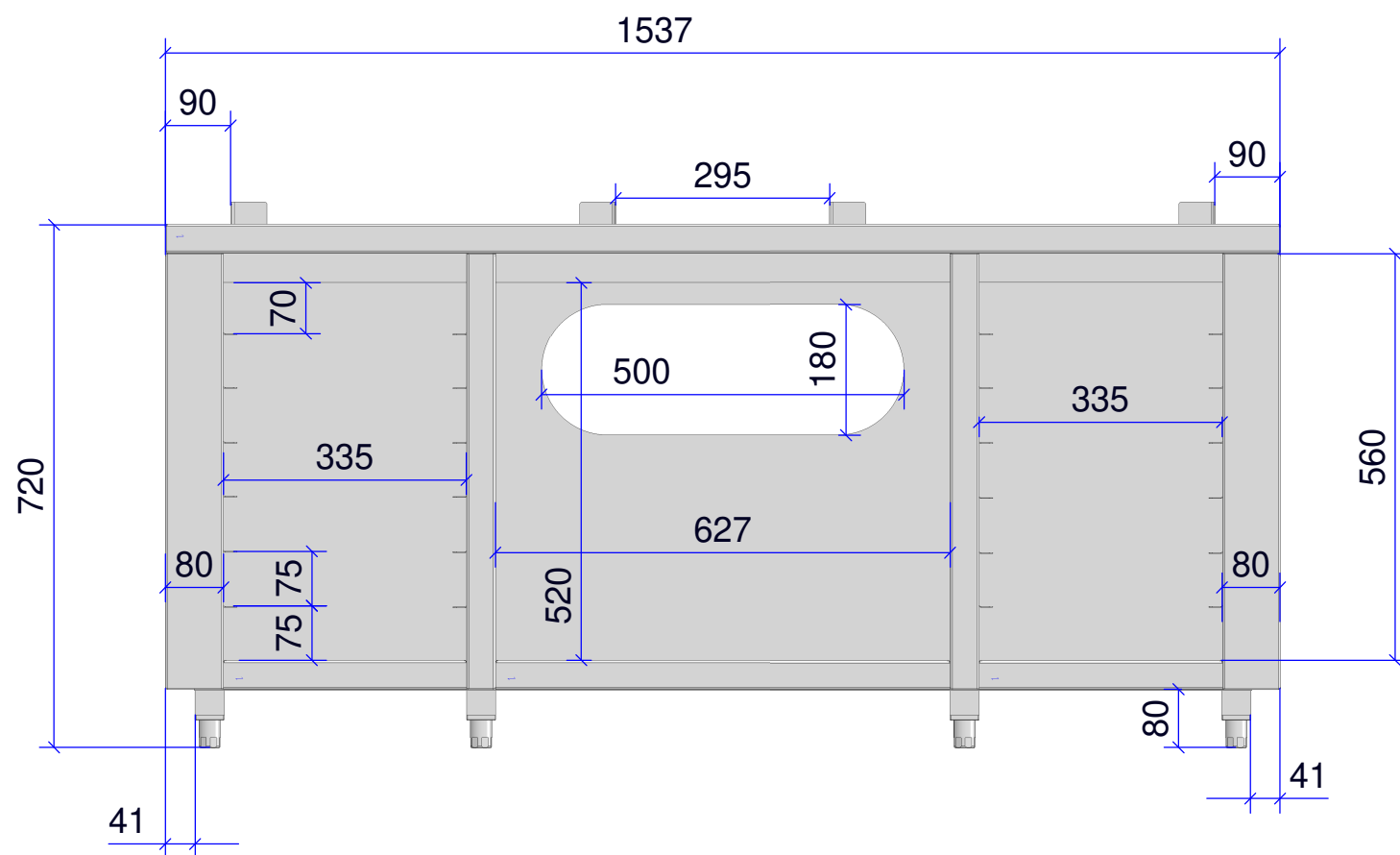
Converge® Multi-Cook Oven Laag Onderstel Uitsparing Voor Warmhoudlade 500-2D / 2DI EN 2X 6 REGALEN (KLP-BASE-CMC2REG)
